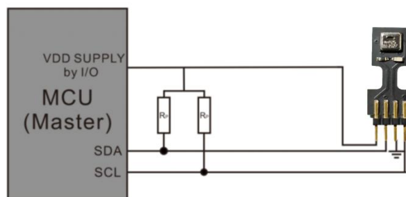
图8 典型的应用电路
