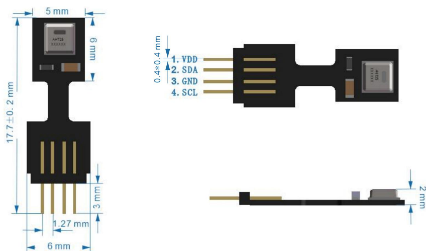
图12 AHT25传感器封装图（单位：mm 未注明公差：0.1mm）
