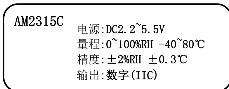
图14. 纸盒上的标签
